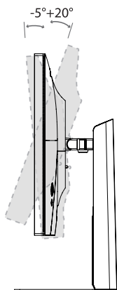
Угол наклона -5^\circ (\pm 2^\circ) - +20^\circ (\pm 2^\circ)
